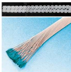
LHC
